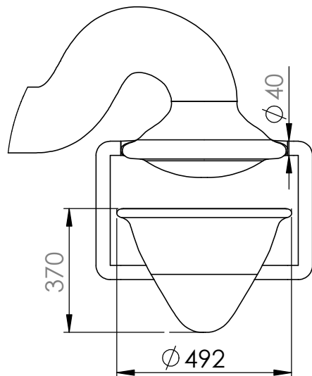
SZCZEGÓŁ A SKALA 1 : 15
