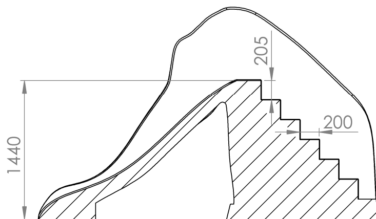
PRZEKRÓJ A-A SKALA 1 : 40
